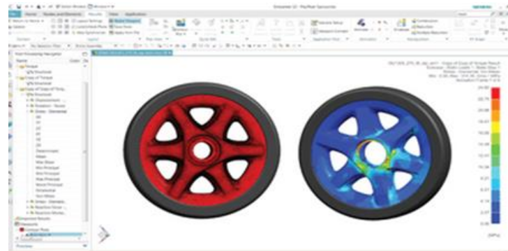
Análisis FEA de las ruedas
